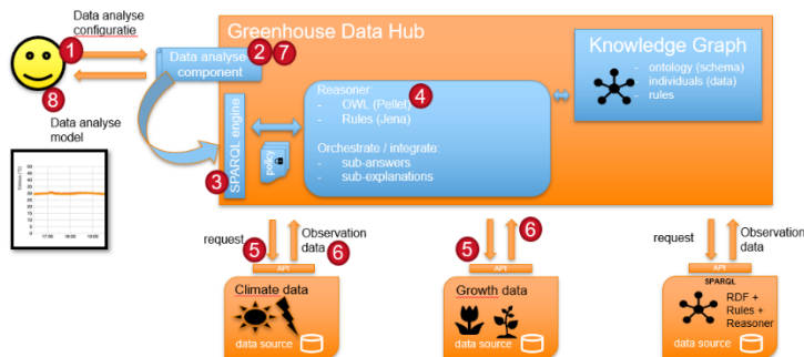
Figuur 2 Data-analyse architectuur.
